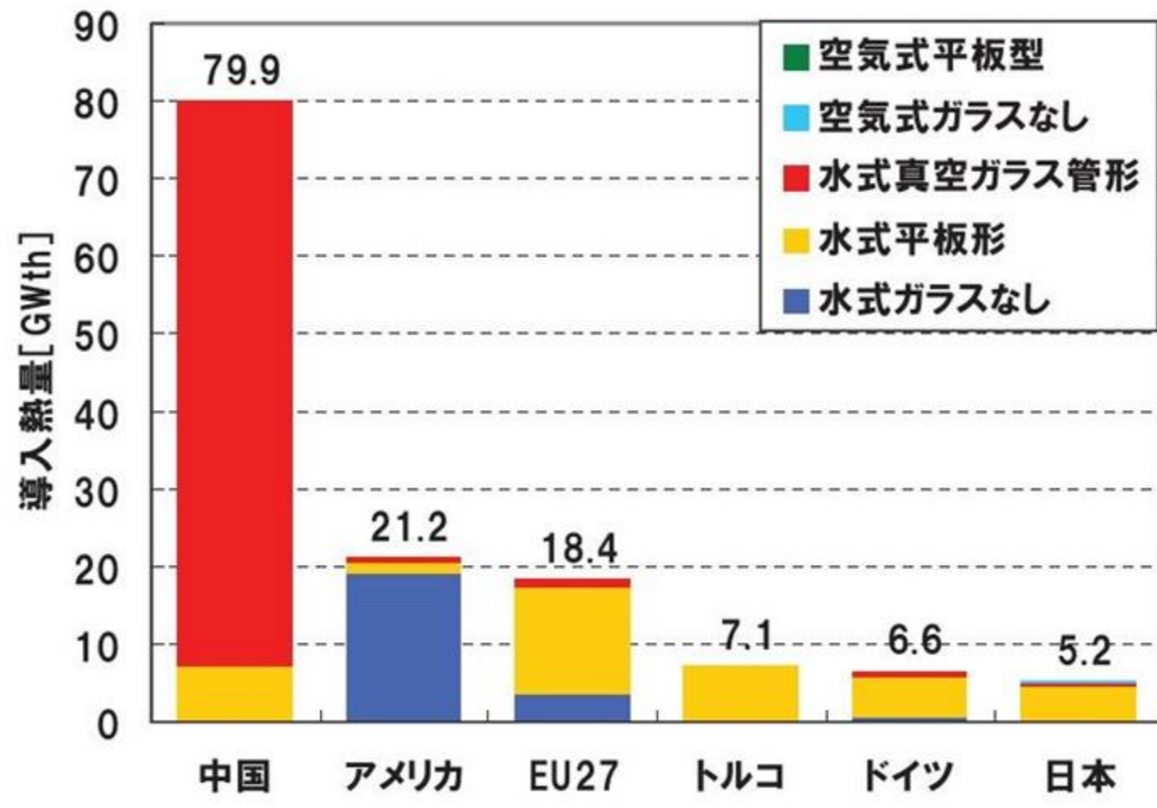
図 太陽熱導入量の比較(2007年) 出所: Solar Heat Worldwide Markets and Contribution to the Energy Supply 2007 (EDITION 2009), IEA Solar Heating & Cooling Programme より作成
